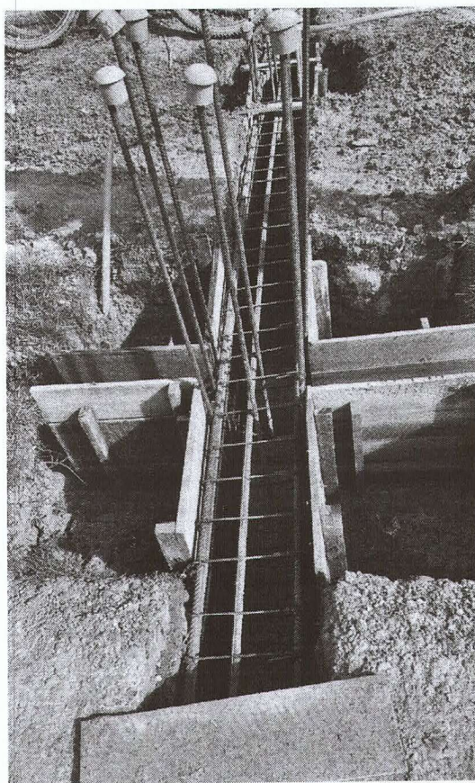
Imagens 04 e 05 – Fundações do Bloco B
