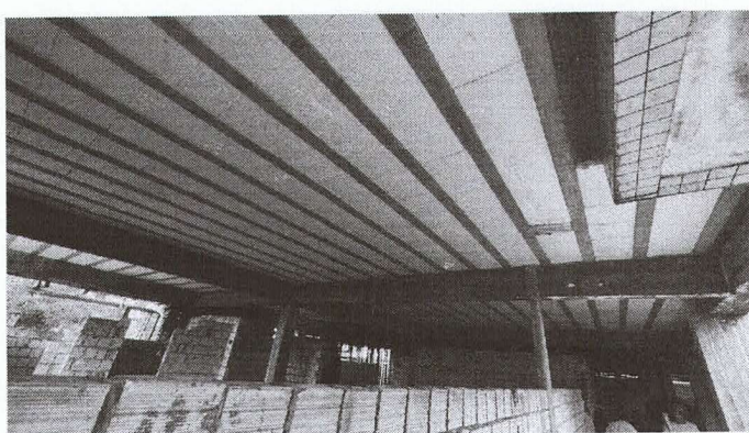
Imagens 01 e 02 – Laje de Cobertura do Bloco A concluída.
