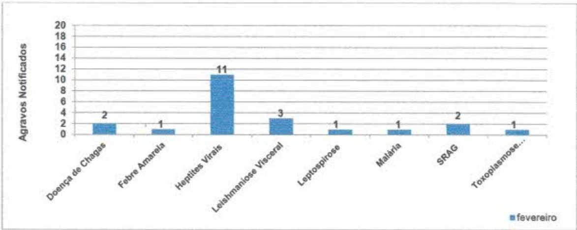
Figura 1: Demonstrativo das notificações realizadas e encaminhadas à Vigilância Epidemiológica Municipal fevereiro de 2024.
