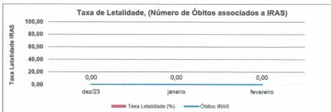
Figura 21: Gráfico demonstrativo da taxa de letalidade associada as IRAS.
